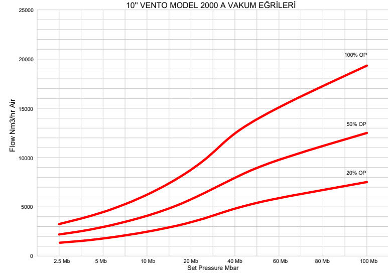
10" VENTO MODEL 2000 A VAKUM EĞRİLERİ
