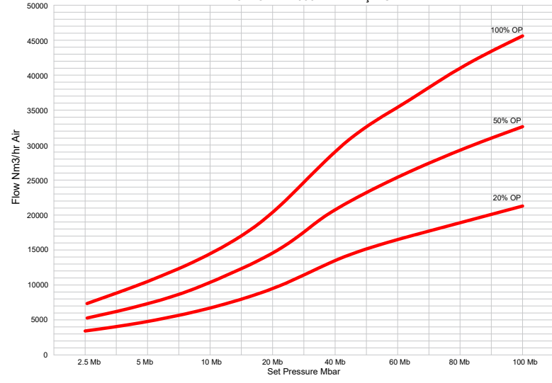
12" VENTO MODEL 2000 A BASINÇ EĞRİLERİ
