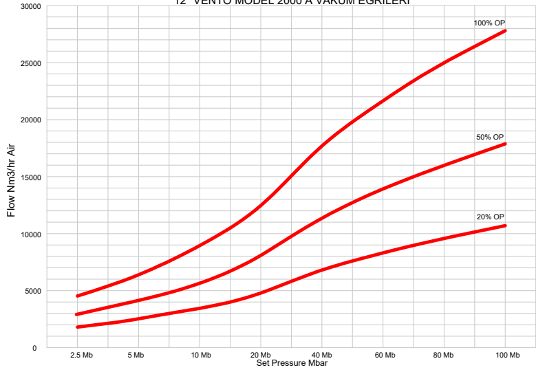
12" VENTO MODEL 2000 A VAKUM EĞRİLERİ
