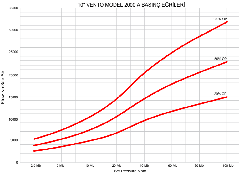
10" VENTO MODEL 2000 A BASINÇ EĞRİLERİ
