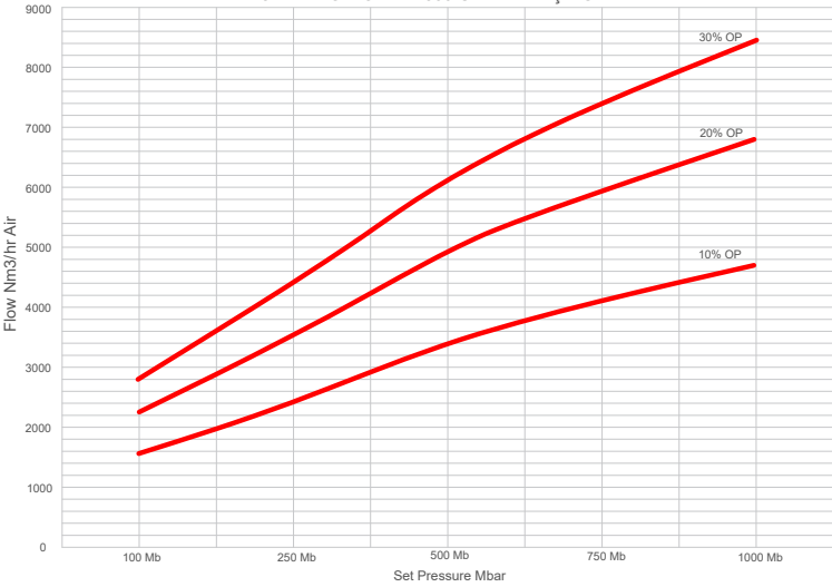
8" VENTO MODEL 2300 CPS BASINÇ EĞRİLERİ
