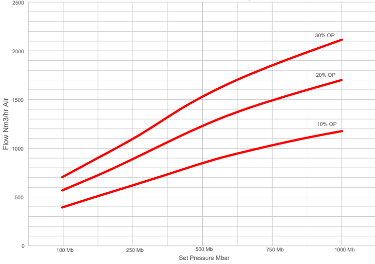
4" VENTO MODEL 2300 CPS BASINÇ EĞRİLERİ
