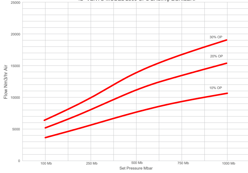
12" VENTO MODEL 2300 CPS BASINÇ EĞRİLERİ
