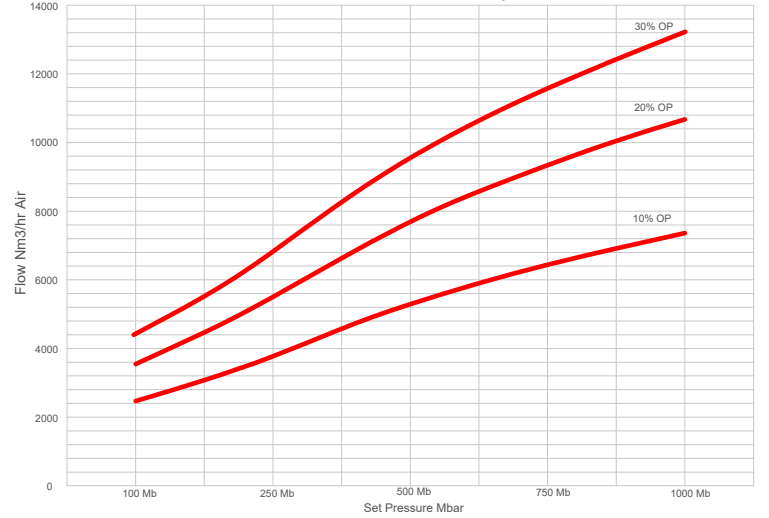
10" VENTO MODEL 2300 CPS BASINÇ EĞRİLERİ
