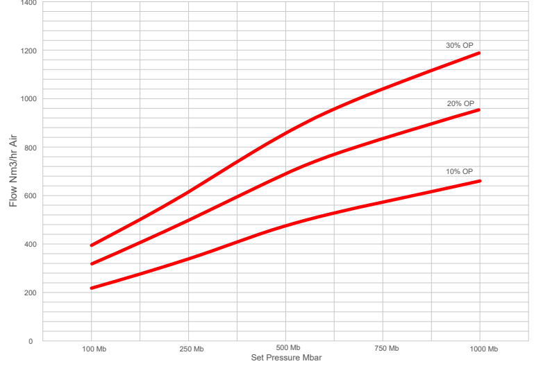
6" VENTO MODEL 2300 CPS BASINÇ EĞRİLERİ
