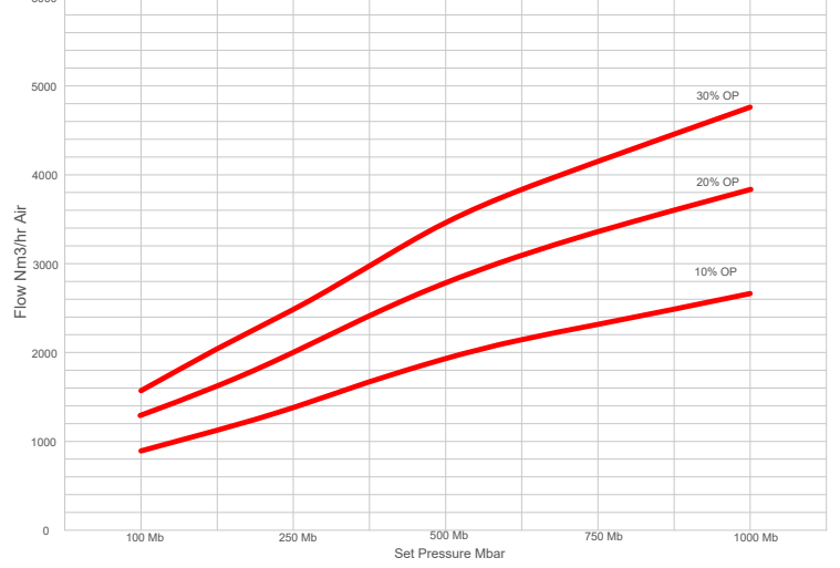
6" VENTO MODEL 2300 CPS BASINÇ EĞRİLERİ
