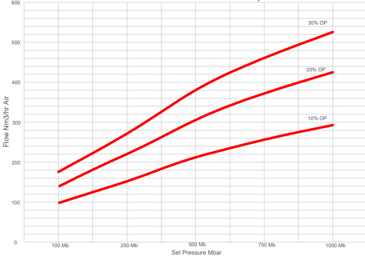
4" VENTO MODEL 2300 CPS BASINÇ EĞRİLERİ
